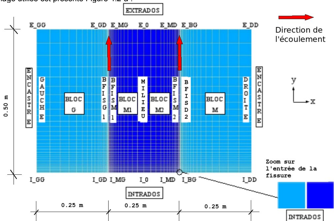
Figure 4.2-a : Maillage complet
