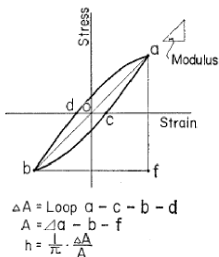
Figure 3.6.5-a: Définition de l'amortissement hystérétique d'après Kokusho []
