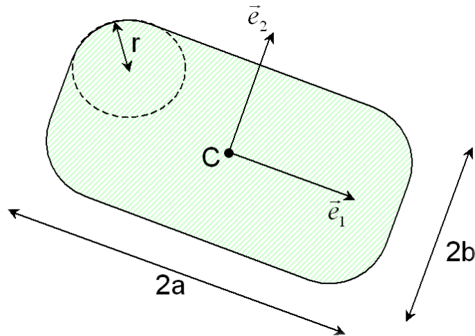
Figure 3.4.3.2-1: schéma d'une fissure/inclusion rectangulaire à coins arrondis
