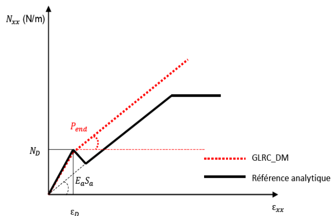
Figure 4.5.1-a: Courbe de traction (GLRC_DM vs Référence) Recalage PENTE = RIGI_ACIER
