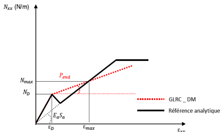
Figure 4.5.1-a: Courbe de traction (GLRC_DM vs Référence) Recalage PENTE = RIGI_ACIER
