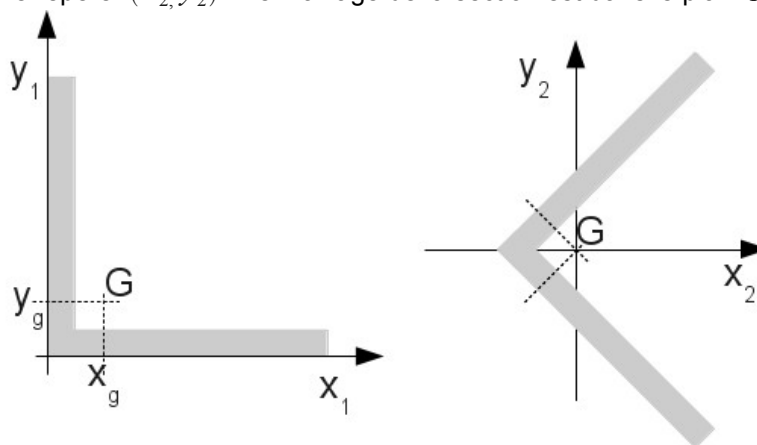
Figure 3.2.1-a : Section cornière.
