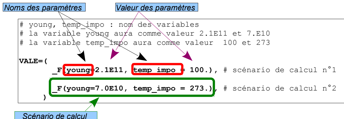
Figure 2.2.1-a: Exemple de Fichier "distr" explicite
