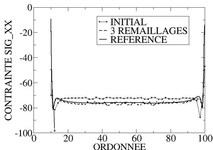
Figure 5.5-c : Profil de contrainte
