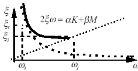
Figure 3.3.1.2-c : allure de l'amortissement de Rayleigh complet.
