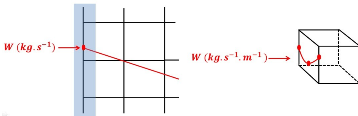
Figure 2.8.4-a : imposition d'un flux à l'embouchure d'une interface cohésive pour un modèle 2D (à gauche) et pour un modèle 3D (à droite).
