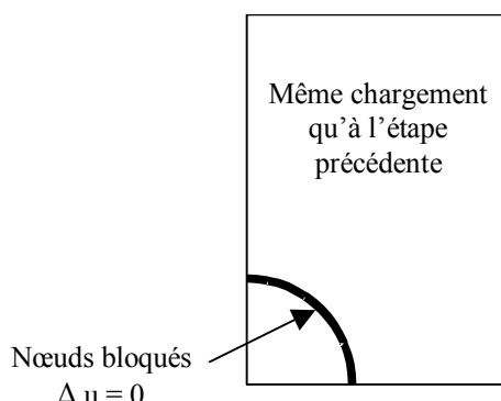
Figure 4.3-a : Blocage des nœuds du bord de la galerie pour y calculer les réactions nodales
