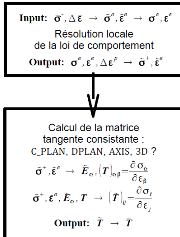
Figure 5.2.4-1: Processus de résolution de la loi de Mohr-Coulomb. Mise en évidence de l'écriture dans les différentes bases de projection.
