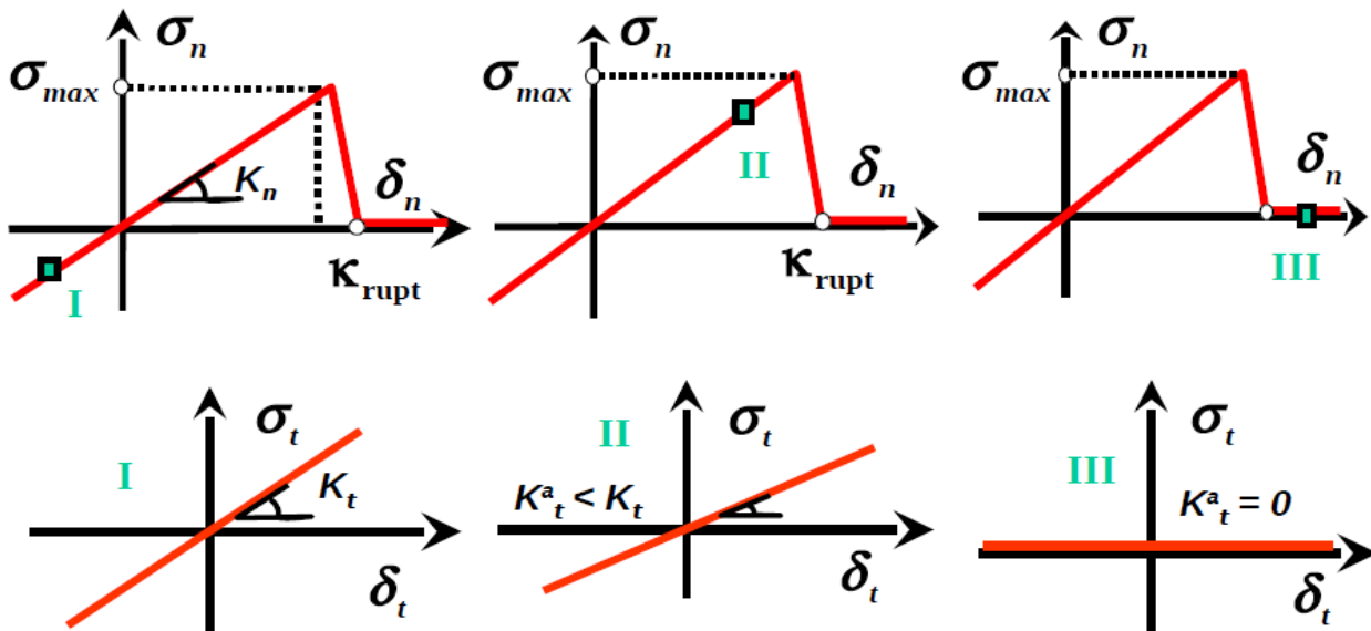
Figure 2.3-3: Illustration du couplage entre le cisaillement et l'ouverture normale de joint : I dans le régime en compression ; II dans le régime d'ouverture partiel ; III dans le régime d'ouverture complète. On note K_t^a \equiv (1 - \delta_n / \kappa_{rupt}^{tan}) K_t
