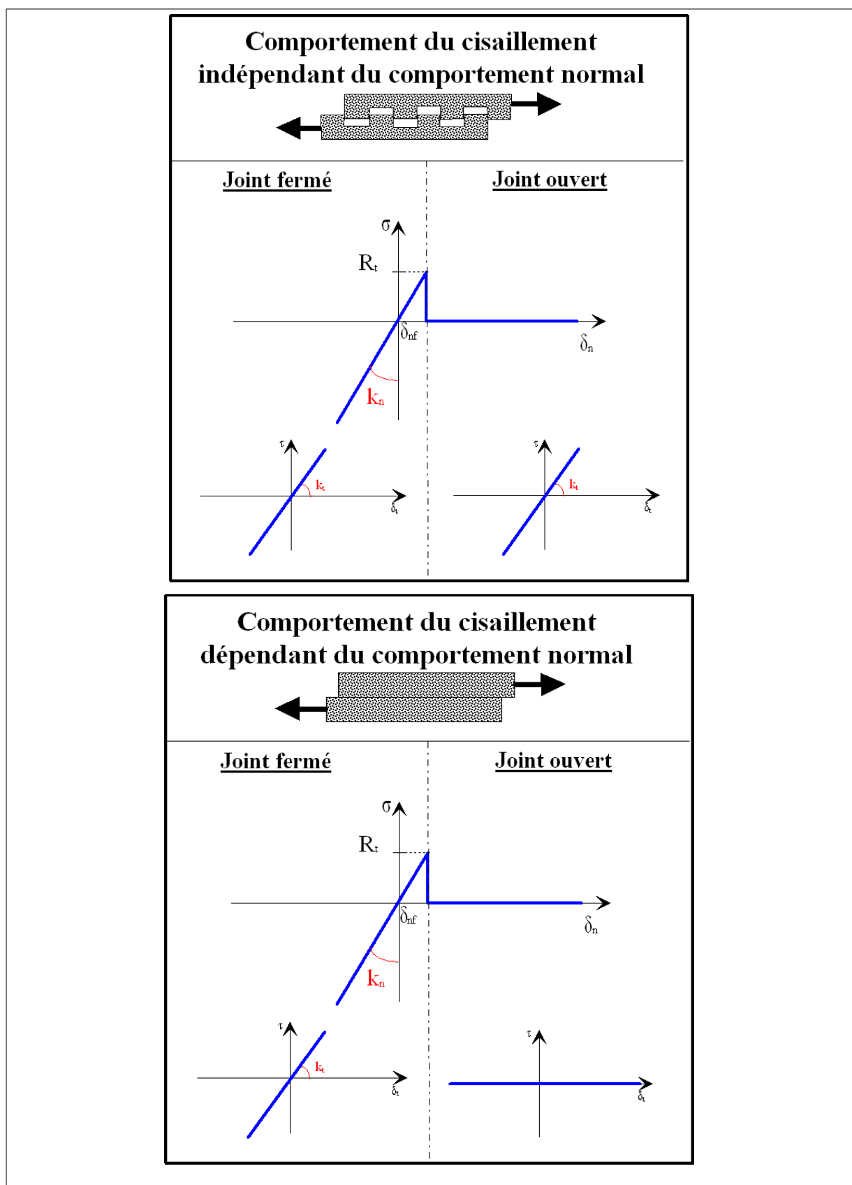
Figure 1.2-1: Comportement normal et tangentiel en fonction de profil de joint
