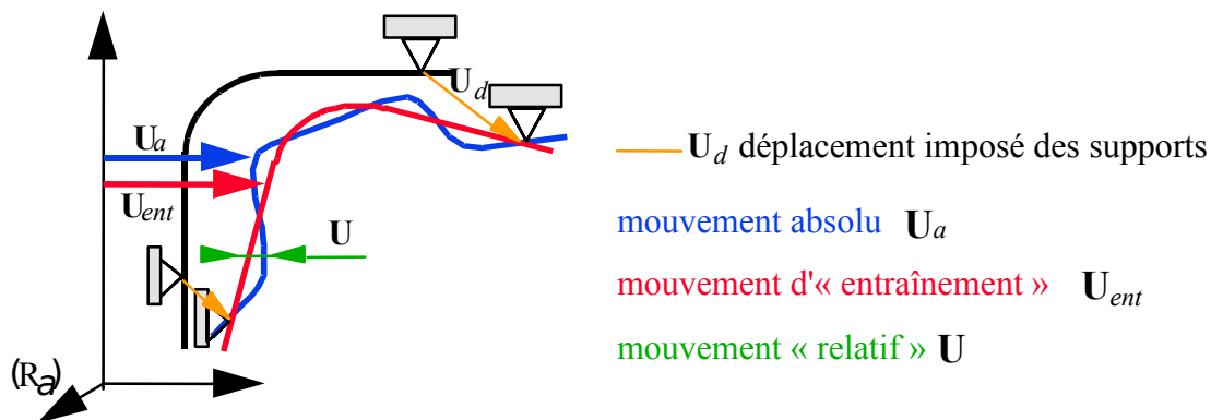
Figure 2.6.1-a : Décomposition du mouvement absolu.
