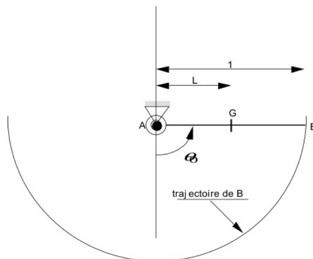
Figure 6-a : Pendule de grande amplitude
