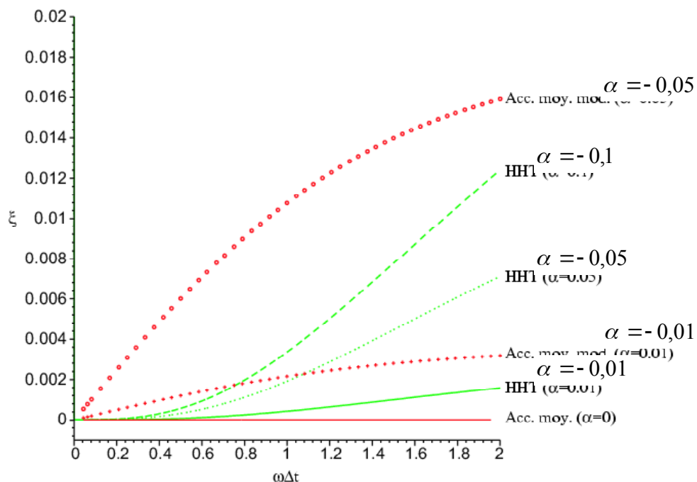
Figure 5.4-a : Taux d'amortissement numérique en fonction du pas de temps du schéma HHT, comparaison avec celui produit par le schéma d'accélération moyenne modifiée, cf. [bib29].
