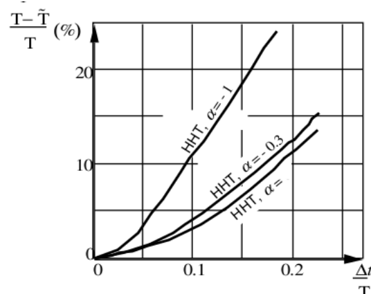
Figure 5.3-b : Erreur relative sur la période en fonction du pas de temps du schéma d'accélération moyenne modifiée
