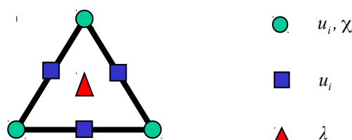
Figure 2.3-a : Discrétisation élément fini du modèle second gradient de dilatation pour les déformations planes
