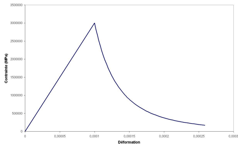
Figure 1 : Réponse contrainte-déformation
