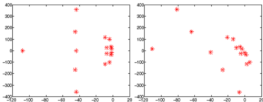
Figure 2.2-1. Exemples du spectre d'un QEP ( n=8 ) d'une modèle simplifié d'enceinte nucléaire [TM01]. Figure de gauche, on est dans le cas n°3 du tableau 2.2-1. Celle de droite, on rajoute à K de l'amortissement hystérétique donc apparaissent des modes dépareillés (cas général n°1).
