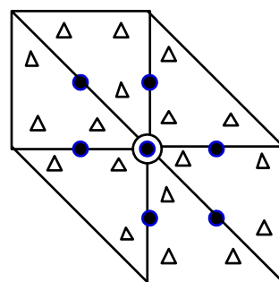
TRIA6
