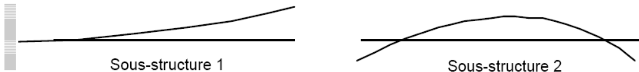
Figure 2.3-c : Modes propres à interfaces libres.
