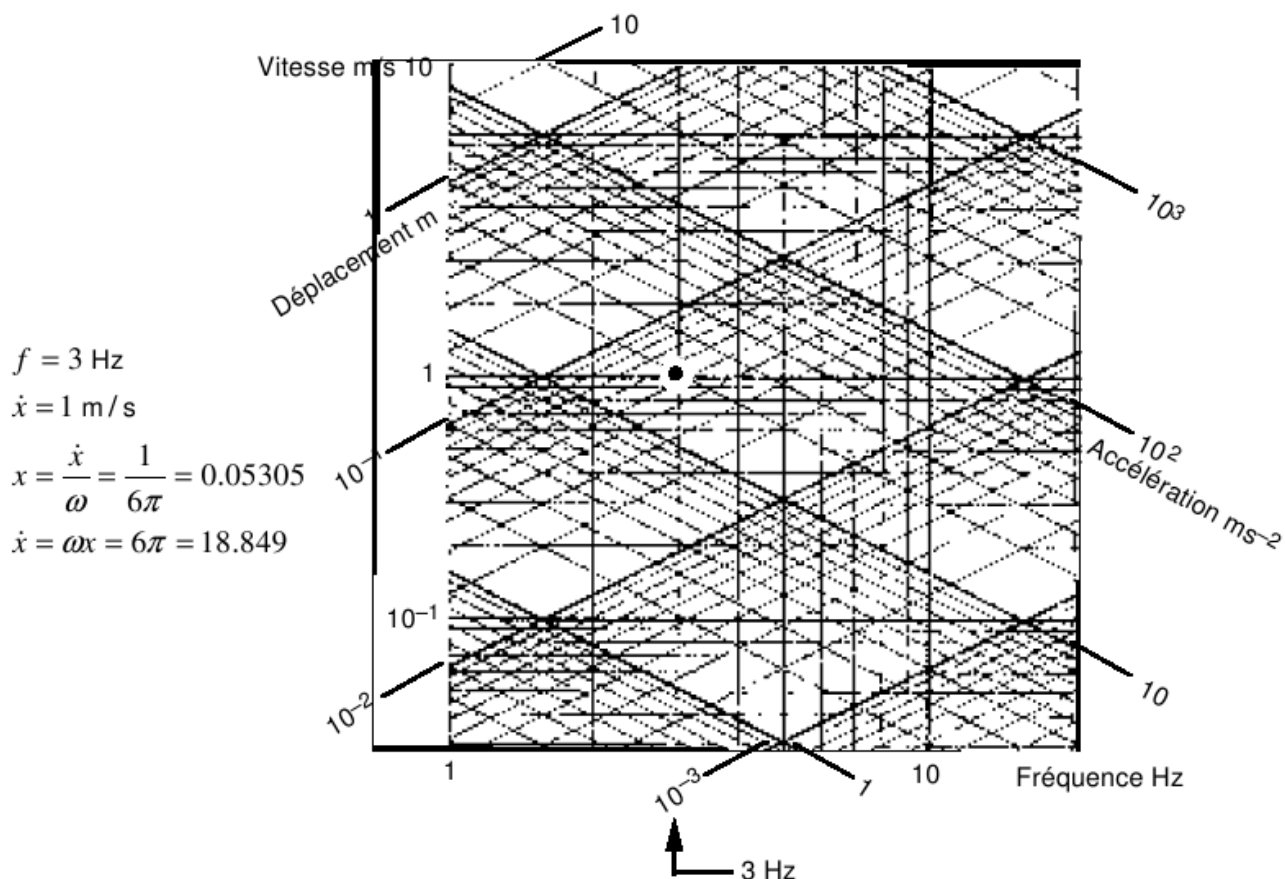
Figure 1.4.1-a : Représentation tri-logarithmique
