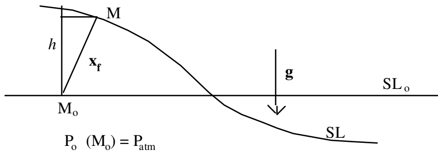
Figure 3.2.1-a : approximation sur la surface libre
