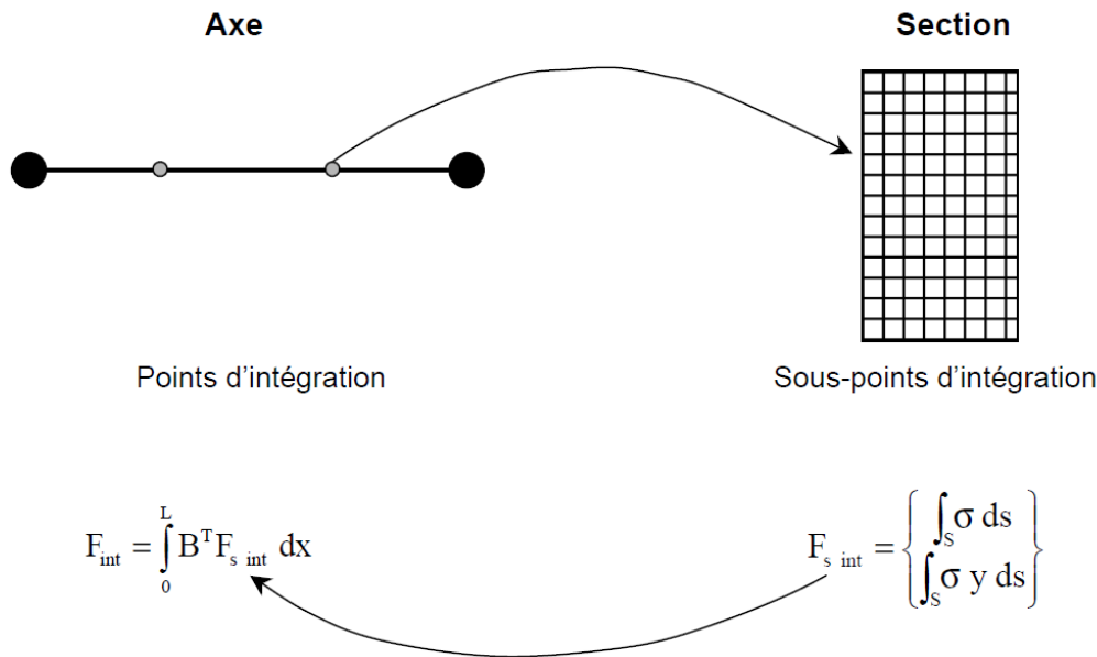
Figure 4.4-a : Poutre multifibre – Calcul de \mathbf{F}_{\text{int}}
