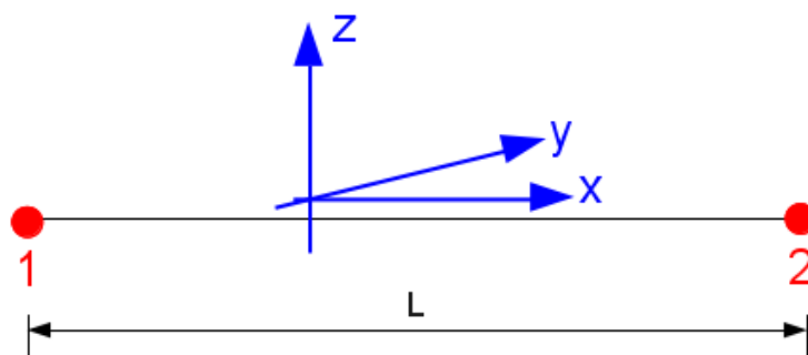
Figure 1-c : Support élément fini d'une modélisation de type poutre multifibre
