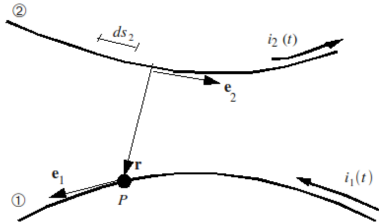
Figure 5 : Disposition de deux conducteurs voisins
