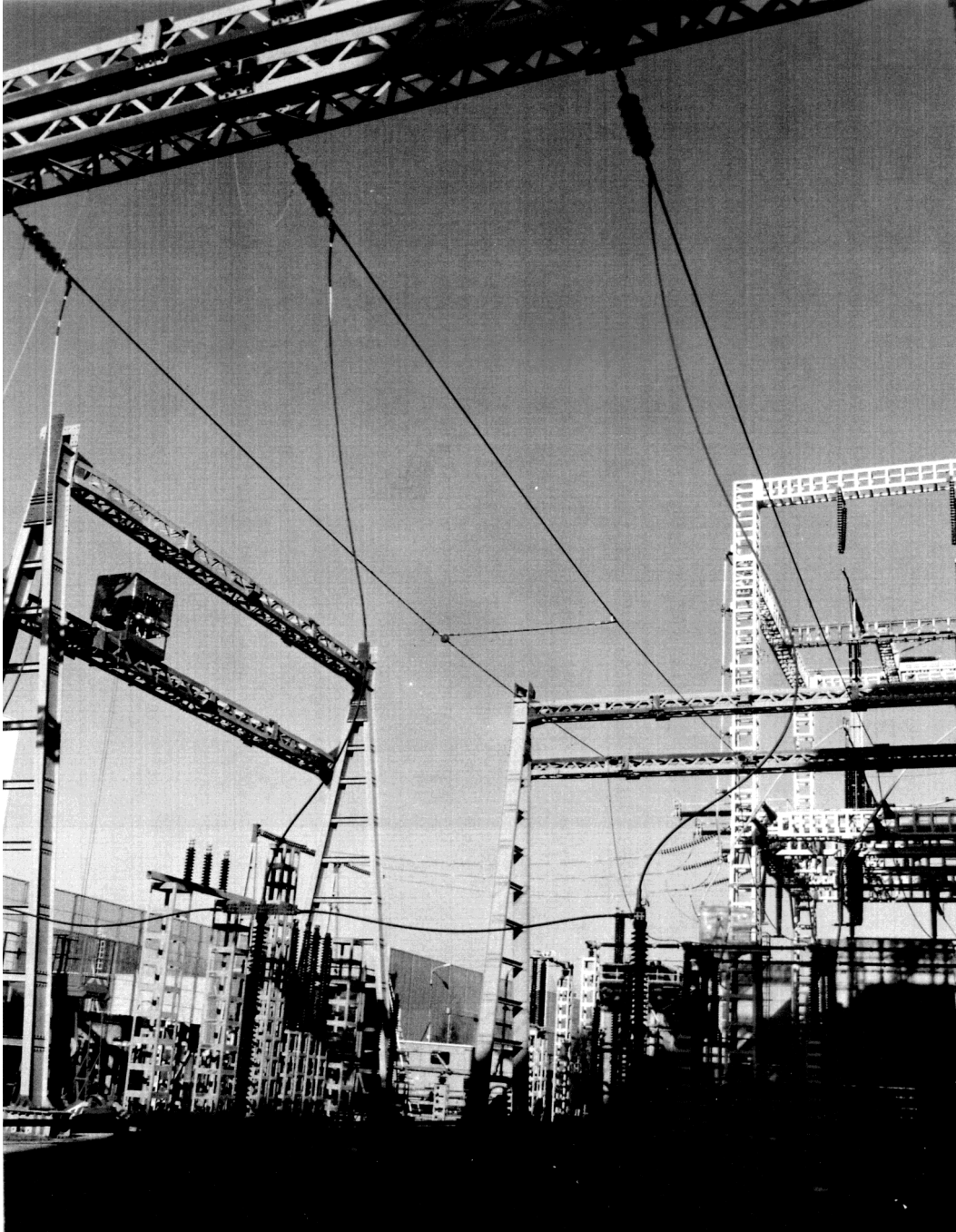
Figure 3 : Vue générale de l'installation d'essais de courts-circuits
