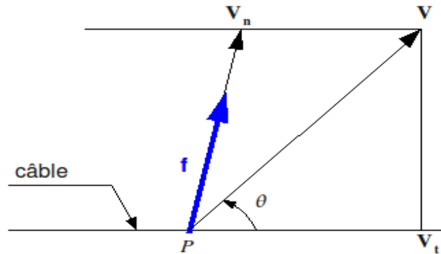
Figure 7 : vitesse du vent au voisinage d'un câble
