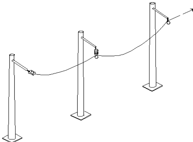
Figure 8 : Pose d'un câble dans un canton à deux portées
