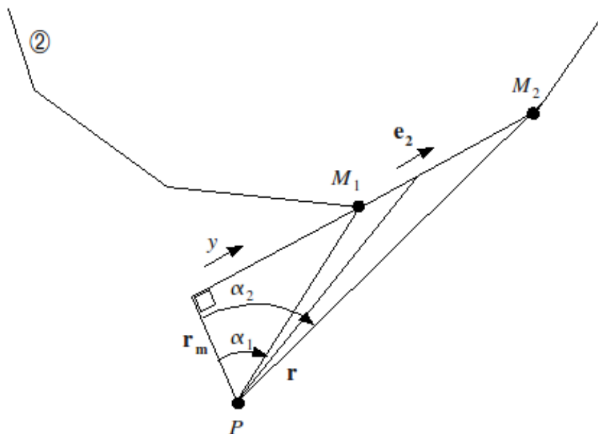
Figure 6 : Force de Laplace induite par un élément rectiligne de conducteur
