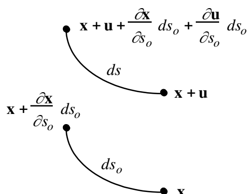
Figure 1 : Tronçon de câble en situations de référence et déplacée
