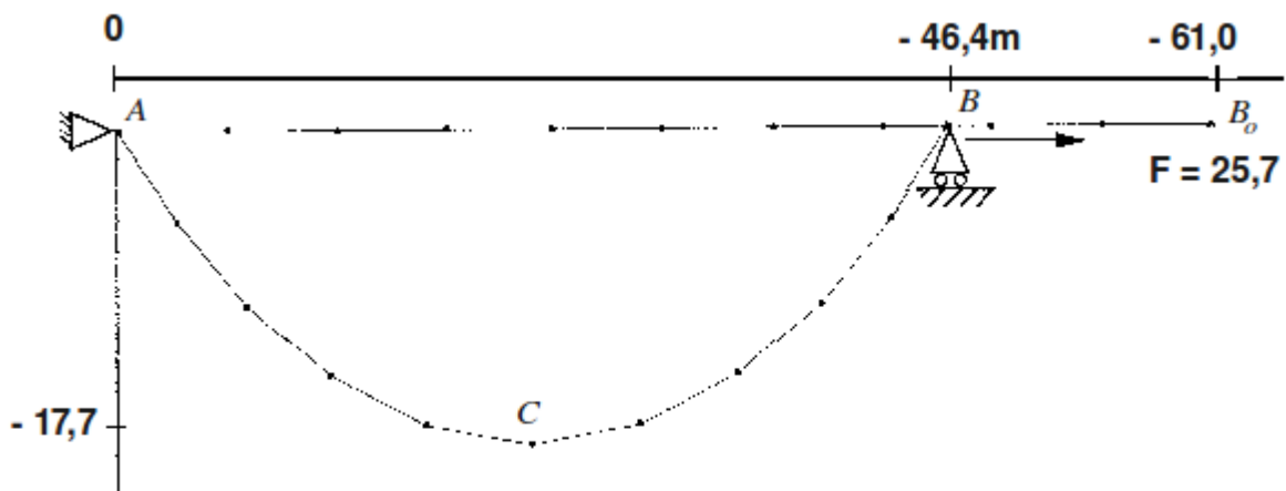
Rigidité extensionnelle (E.A) : 4,45 \times 10^5 N, Poids linéique : 1,46 N/m Figure 2 : Équilibre d'un câble pesant soumis à une tension horizontale
