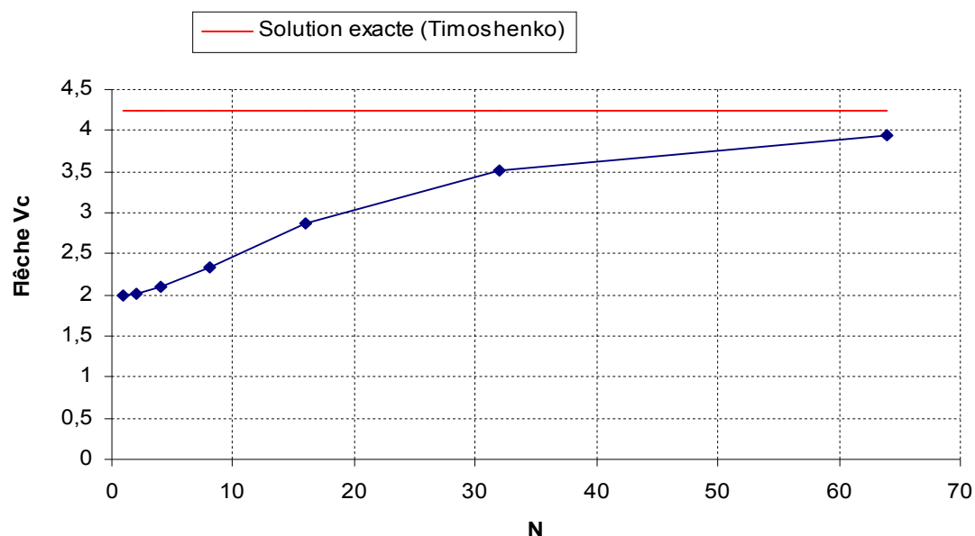
Figure 1.1-b : convergence de l'élément QUAD4 en déformation planes
