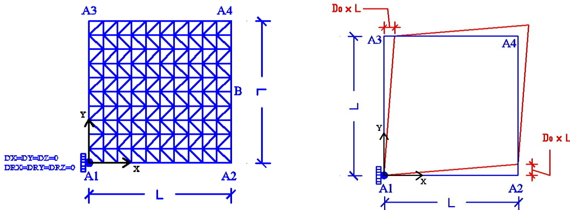
Figure 6.1-a: Maillage et conditions aux limites.
