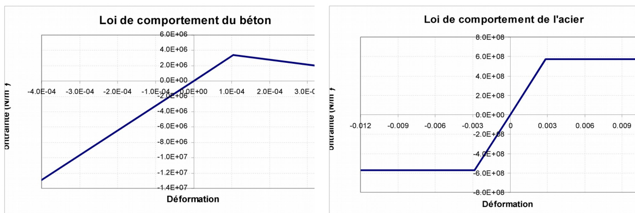
Figure 2.2-a: courbes rationnelles des matériaux (pour modèle multicouche).
