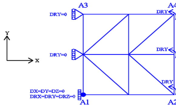
Figure 4.1-a: maillage et conditions aux limites
