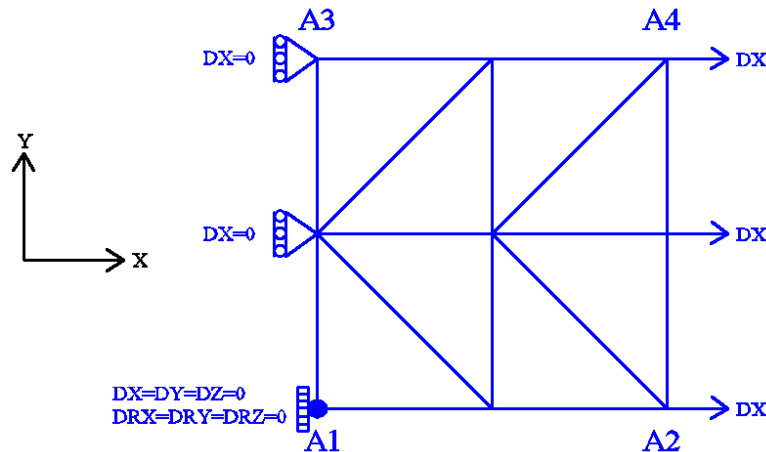
Figure 3.1-a: maillage et conditions aux limites.
