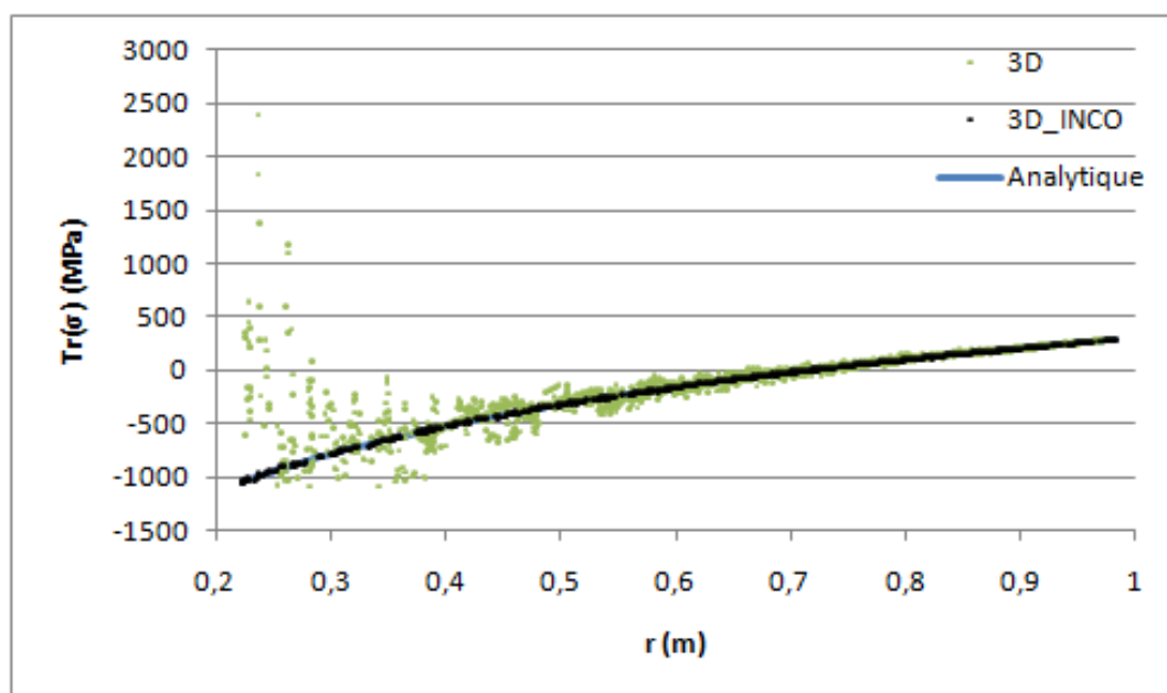
Figure a : Trace des contraintes en Mpa pour les formulations 3D, 3D_INCO et la solution analytique
