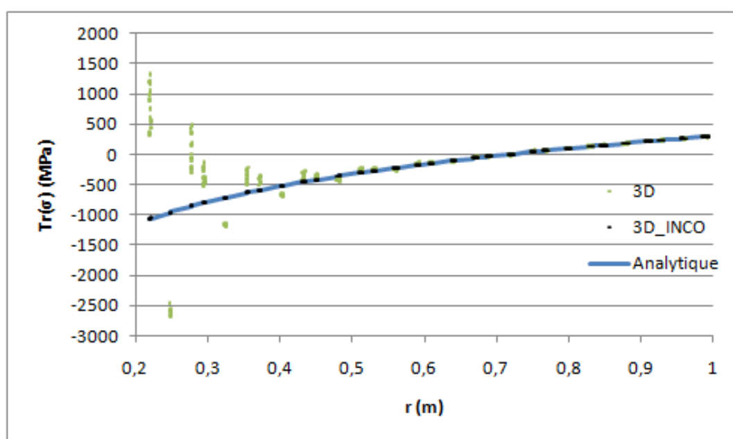
Figure 5.4-a : Trace des contraintes en MPa pour les formulations 3D, 3D_INCO et la solution analytique
