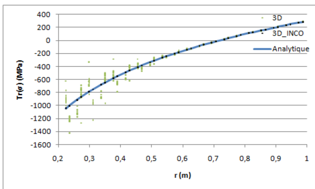
Figure 7.4-a : Trace des contraintes en Mpa pour les formulations AXIS , AXIS_INCO et la solution analytique
