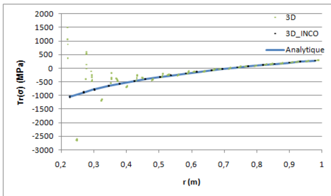
Figure 3.4-a : trace des contraintes en Mpa pour les formulations 3D, 3D_INCO et la solution analytique
