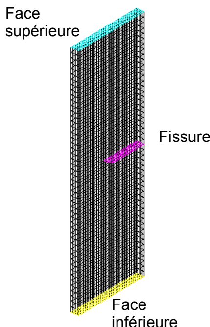
Figure 2.1-a : Maillage fissuré
