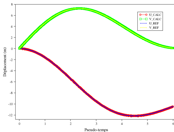
Déplacements U et V en fonction du pseudo-temps
