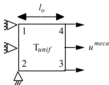
Figure 1.3-1: Conditions limites et chargement
