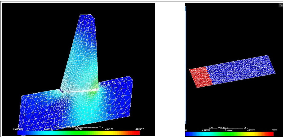
Figure 6.3 : Contraintes sur le barrage et la partie du joint en glissement (en rouge)
