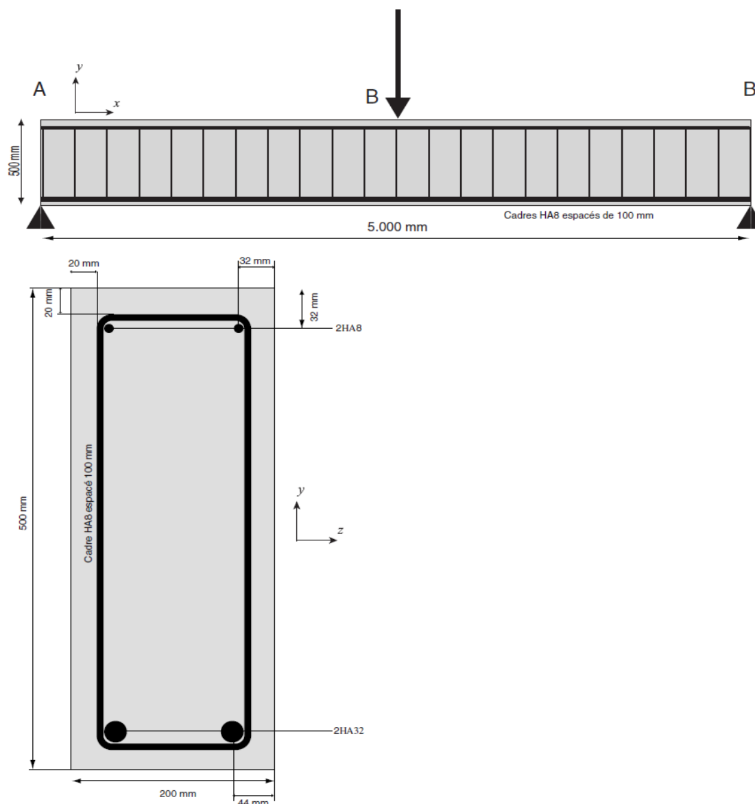
Figure 1.1-a : Plan de la poutre.
