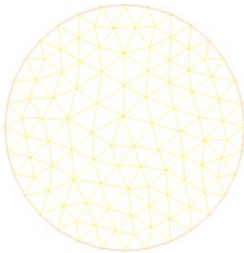
111 nœuds, 188 TRIA3
