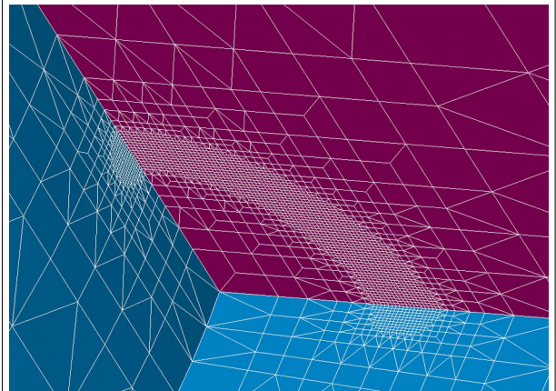
Figure 4.2-2: modélisation B, vue en coupe longitudinale du maillage sain raffiné au niveau de la position de la fissure
