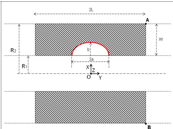
Figure 1.1-2: vue en coupe longitudinale (plan z=0 contenant les lèvres et le front de fissure)
