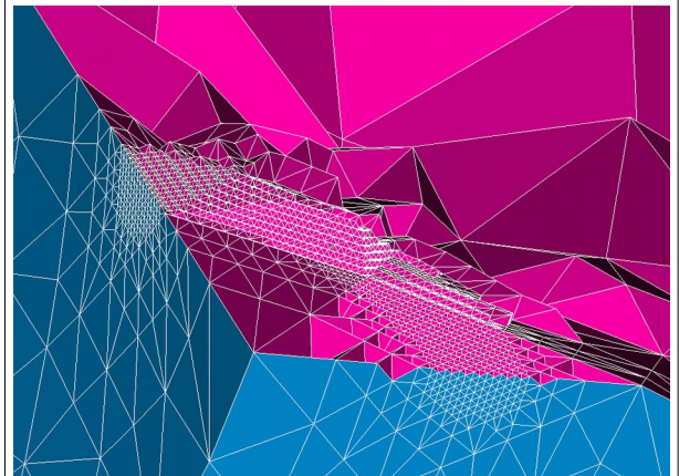
Figure 5.2-2: modélisation C, vue en coupe longitudinale du maillage sain raffiné au niveau de la position de la fissure
