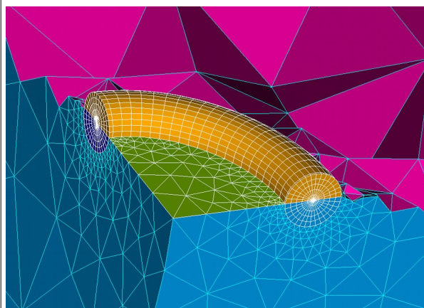
Figure 3.2-2: modélisation A, maillage fissuré, tore en front de fissure
