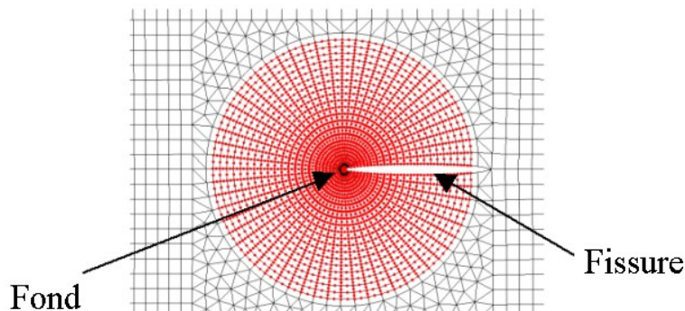
Figure 2.2 : Maillage : zoom sur la fissure.
