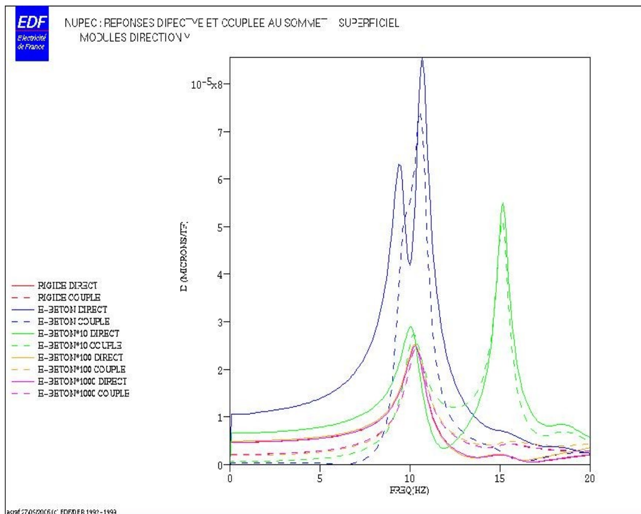
Figure 5-b : Comparaison des modules des réponses directe et couplée à l'excitation harmonique entre cas rigide et cas souple avec augmentation du module de la fondation de liaison dans la direction Y .
