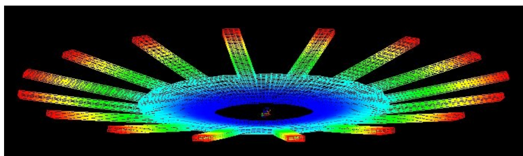
Mode 1 : 31.4503 Hz
