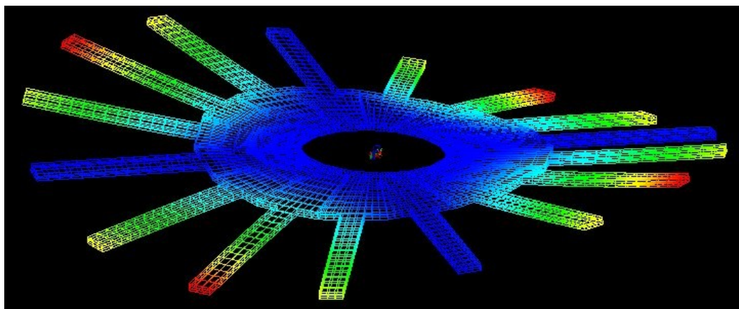
Mode 1 : 33.4833 Hz
