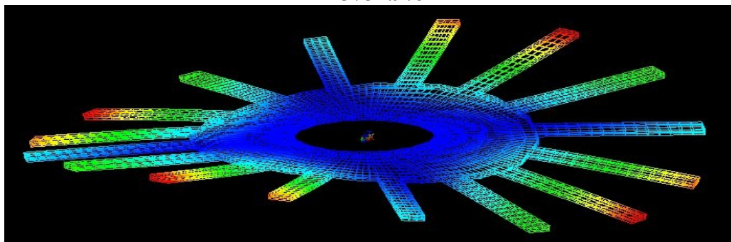
Mode 4 : 33.4833 Hz
