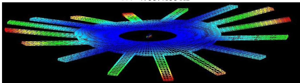
Mode 5 : 33.4833 Hz
