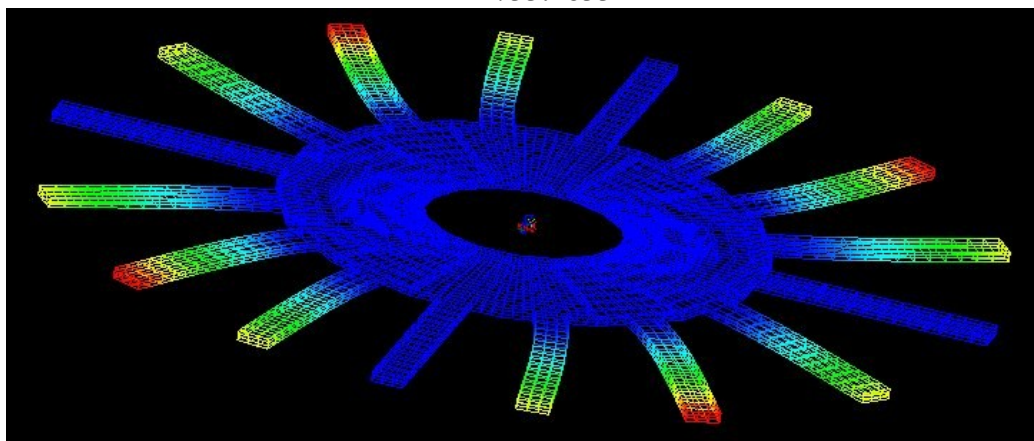
Mode 3 : 44.8997 Hz
