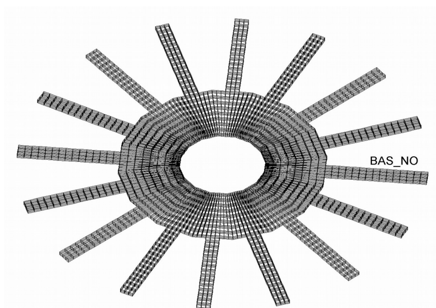
Figure 3.1. Maillage de la modélisation A
