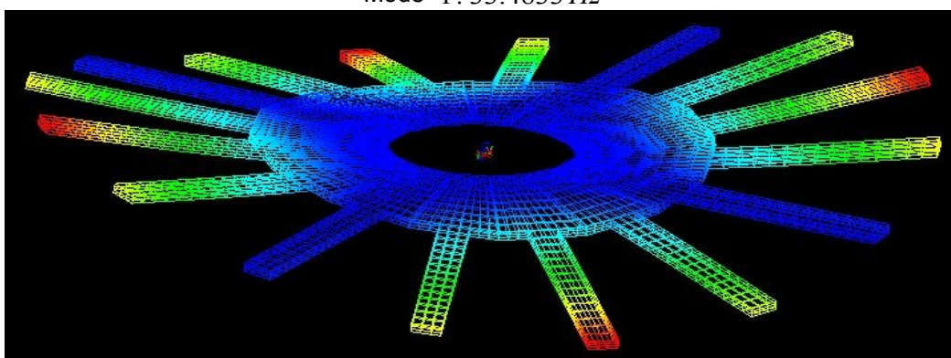
Mode 2 : 33.4833 Hz
