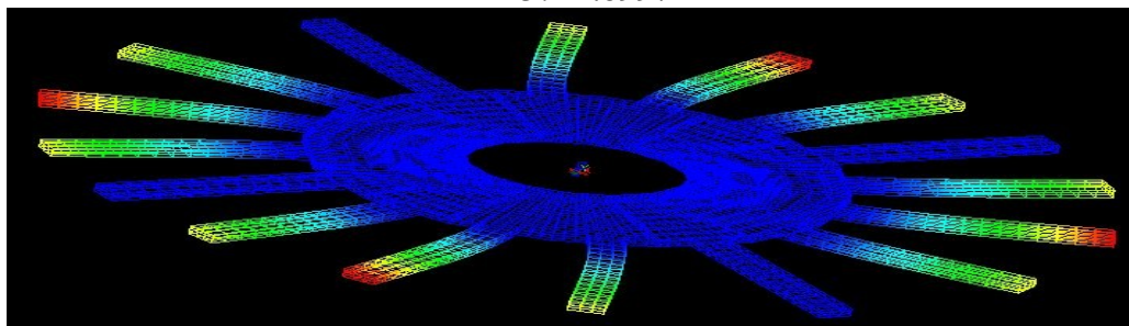
Mode 4 : 44.8997 Hz
