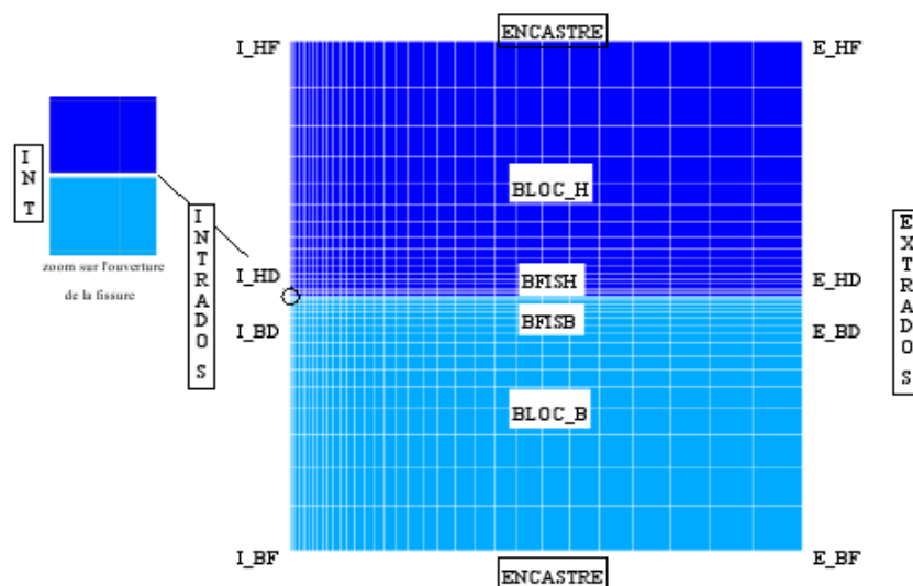
Figure 3.2-a : Maillage complet
