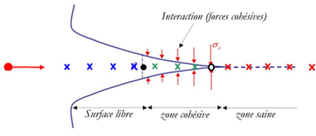
Figure 1 : Schéma de la fissure cohésive et de ses points de Gauss.
