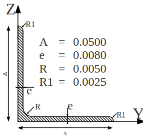
Figure 4.1.1-a : Cornière à ailes égales 50x50x8.
