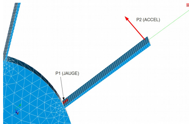
Image 3.2-2: mesure des vibrations d'une ailette à l'aide d'une jauge et d'un accéléromètre.
