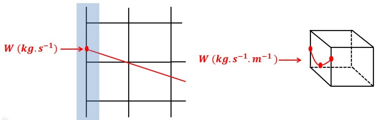
Figure 2.8.4-a : imposition d'un flux à l'embouchure d'une interface cohésive pour un modèle 2D (à gauche) et pour un modèle 3D (à droite).
