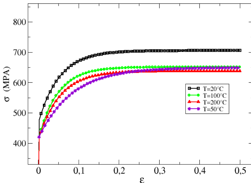
Courbes de traction
