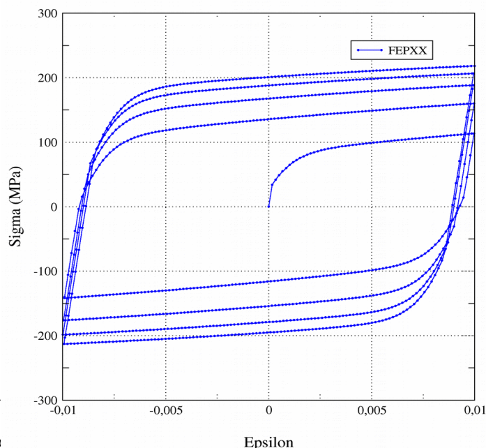
Essai cyclique DEPS=+/-1%
