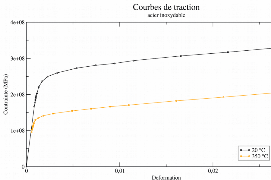
Figure 2.3.1-c . Courbes de traction jusqu'à 3 % de déformation
