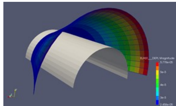
Maillage quadrangles avec une déformée amplifiée
