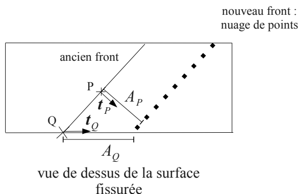
Figure 6.3-c: Avancée de fissure aux points extrémités.
