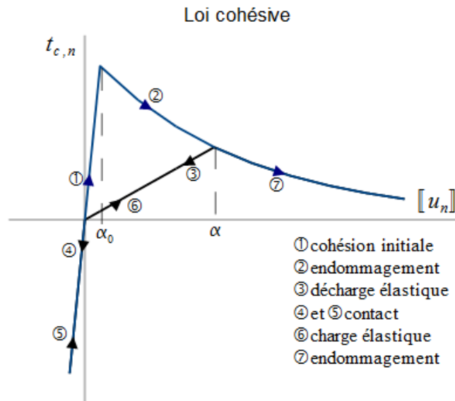
Figure 2.2.1-1: Evolution de la force de cohésion normale en fonction du saut de déplacement.
