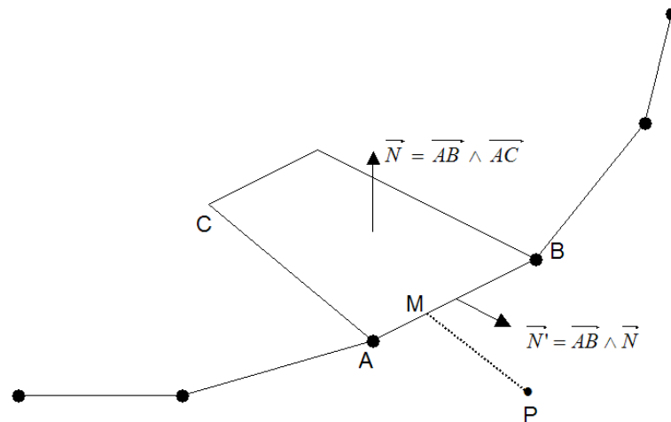
Figure 2.2.2-1 : Calcul de la level set tangente
