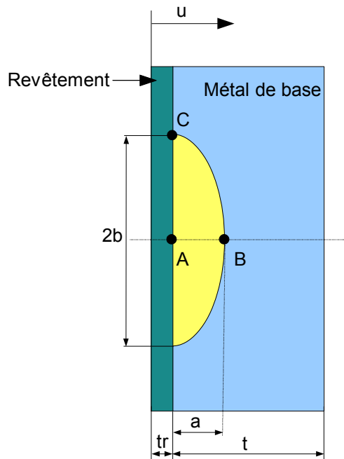
Figure 3.1-a : Défaut semi-elliptique
