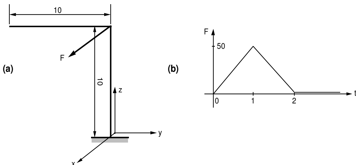
Figure 13.4-a : Potence soumise à une force dynamique perpendiculaire à son plan
