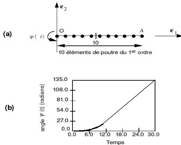
Figure 13.5-a : Bras de robot soumis à une rotation imposée.
