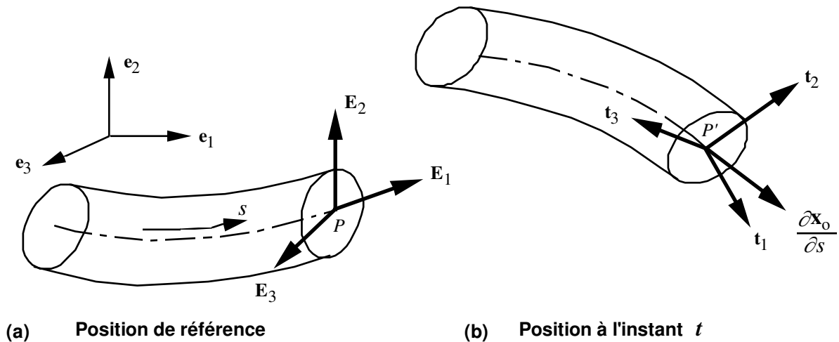
Figure 3-a : Évolution d'un tronçon de poutre
