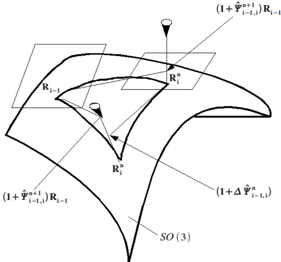
Figure A6-a : Représentation des opérateurs intervenant dans la rotation des sections. : symbole de la projection exponentielle
