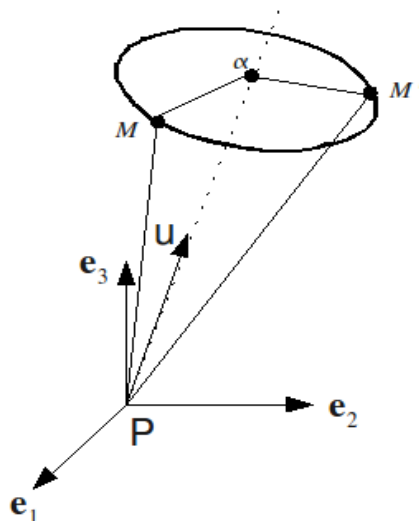
Figure 4.1-a : Représentation d'une rotation finie
