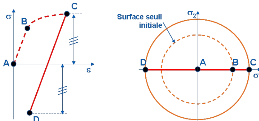
Figure 1.8-1 : Écroissage isotrope
