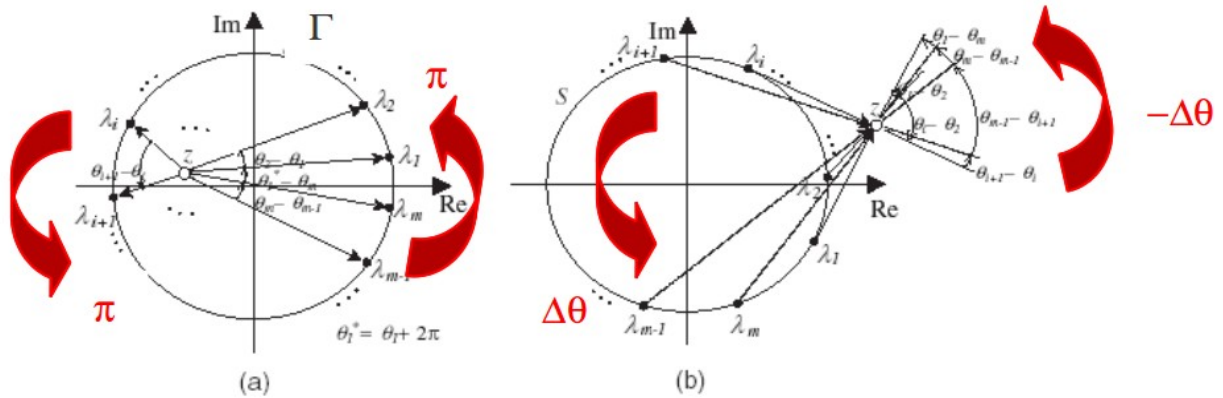
Figure 2.3 Fonctionnement des méthodes de type 'Argument Principal' (extrait de [JHKL03]) décortiqué sur un problème modèle. Il comporte une seule valeur propre simple z et un contour \Gamma de type cercle. Dans le cas (a), le contour entoure cette valeur propre, dans le cas (b), elle lui est extérieure.
