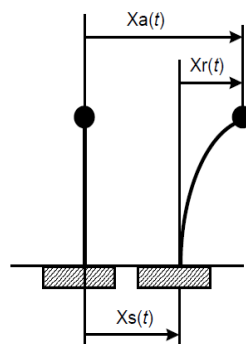
Figure 3.2.2-a : cas « mono-appui ».
