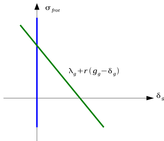
Figure 4-1: Interprétation graphique de l'intégration de la loi d'adhérence parfaite
