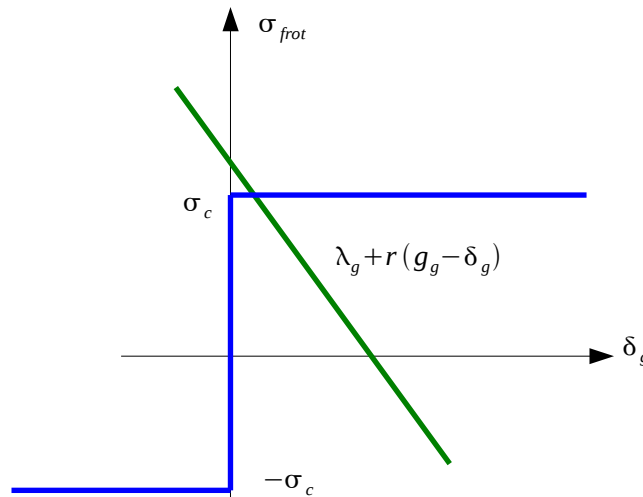
Figure 4-3: Interprétation graphique de l'intégration de la loi de frottement BPEL
