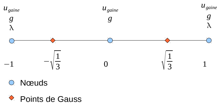
Figure 2-1: discrétisation de l'élément CABLE_GAINE
